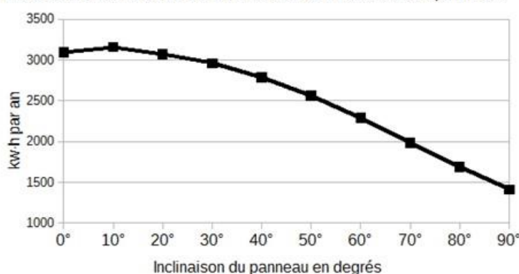
Production annuelle d'électricité en fonction de l'inclinaison des panneaux
